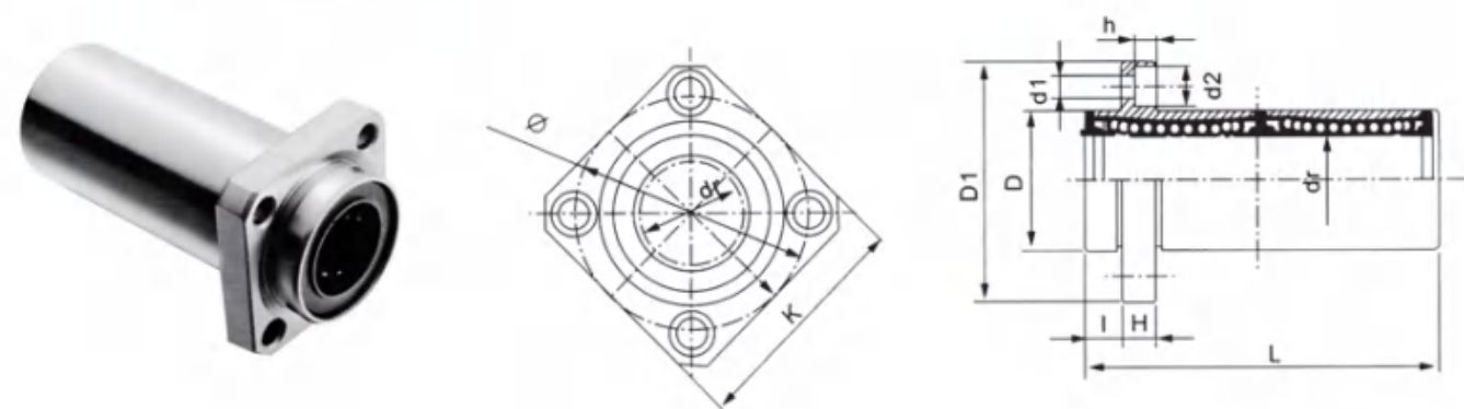
中型导向方法兰型直线轴承 SLMKP □ RUU Series
